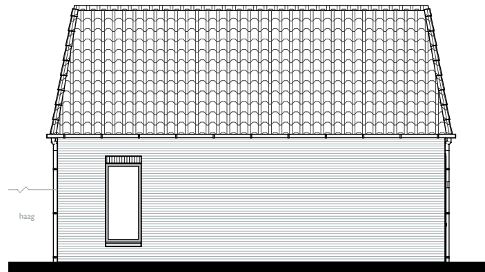
45 Linkergevel (noord)
