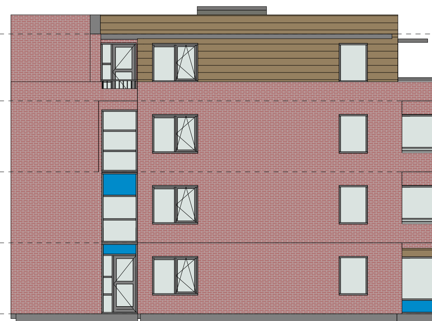
rechtgevel
