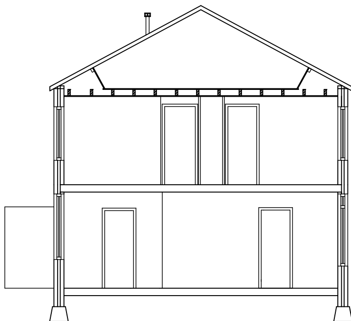
DOORSNEDE WONING
