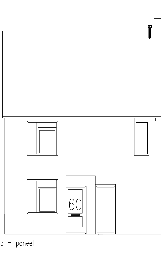
VORGEVEL
